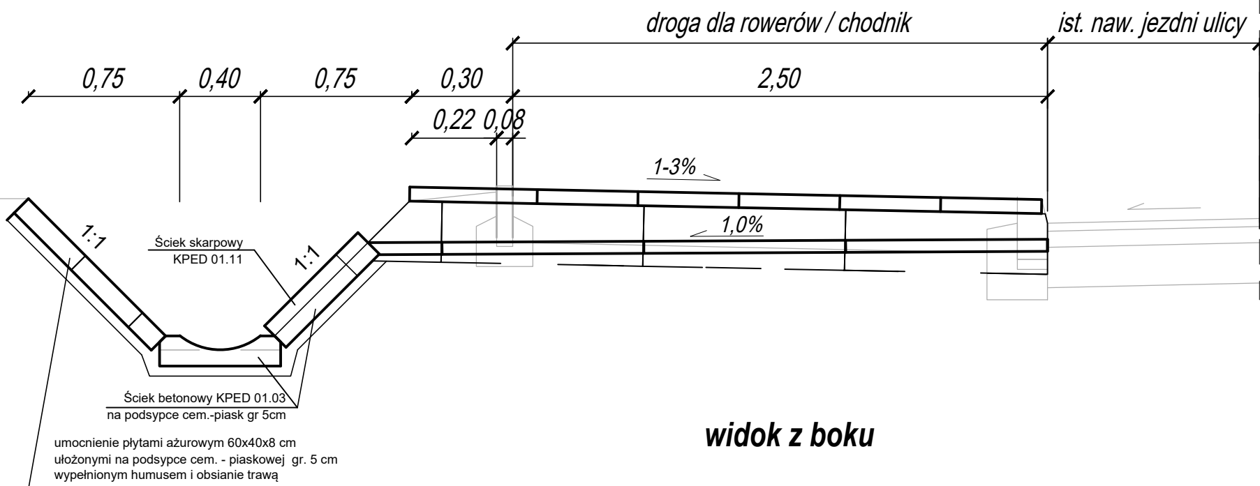
przekrój podłużny
